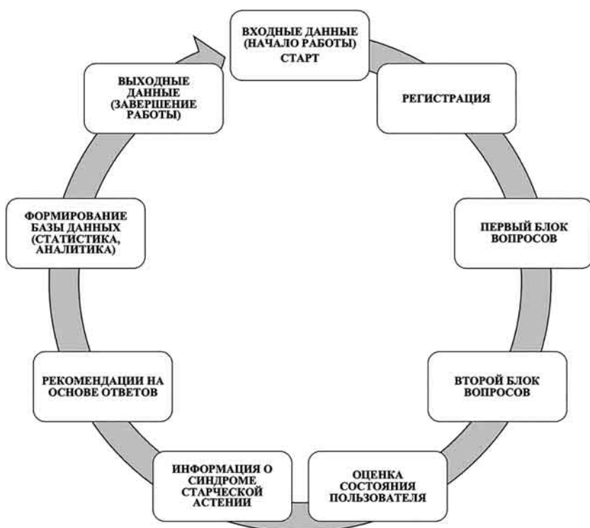
Рис. 1. Алгоритм работы чат-бота для скрининга синдрома старческой астении.
